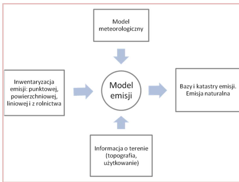
Rysunek 8. Schemat modelowania emisji zanieczyszczeń
