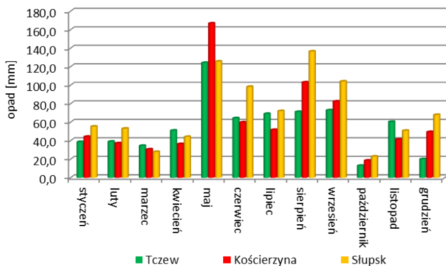
Rysunek 53. Przebieg średnich miesięcznych sum opadów atmosferycznych na wybranych stanowiskach w województwie pomorskim w 2013 r.
