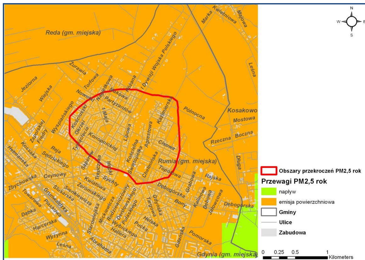
Rysunek 30. Przeważający typ emisji w stężeniach pyłu zawieszonego PM_{2,5} o okresie uśredniania wyników rok w strefie pomorskiej w 2013 r., Rumia – PM13SpoPM2,5a02
