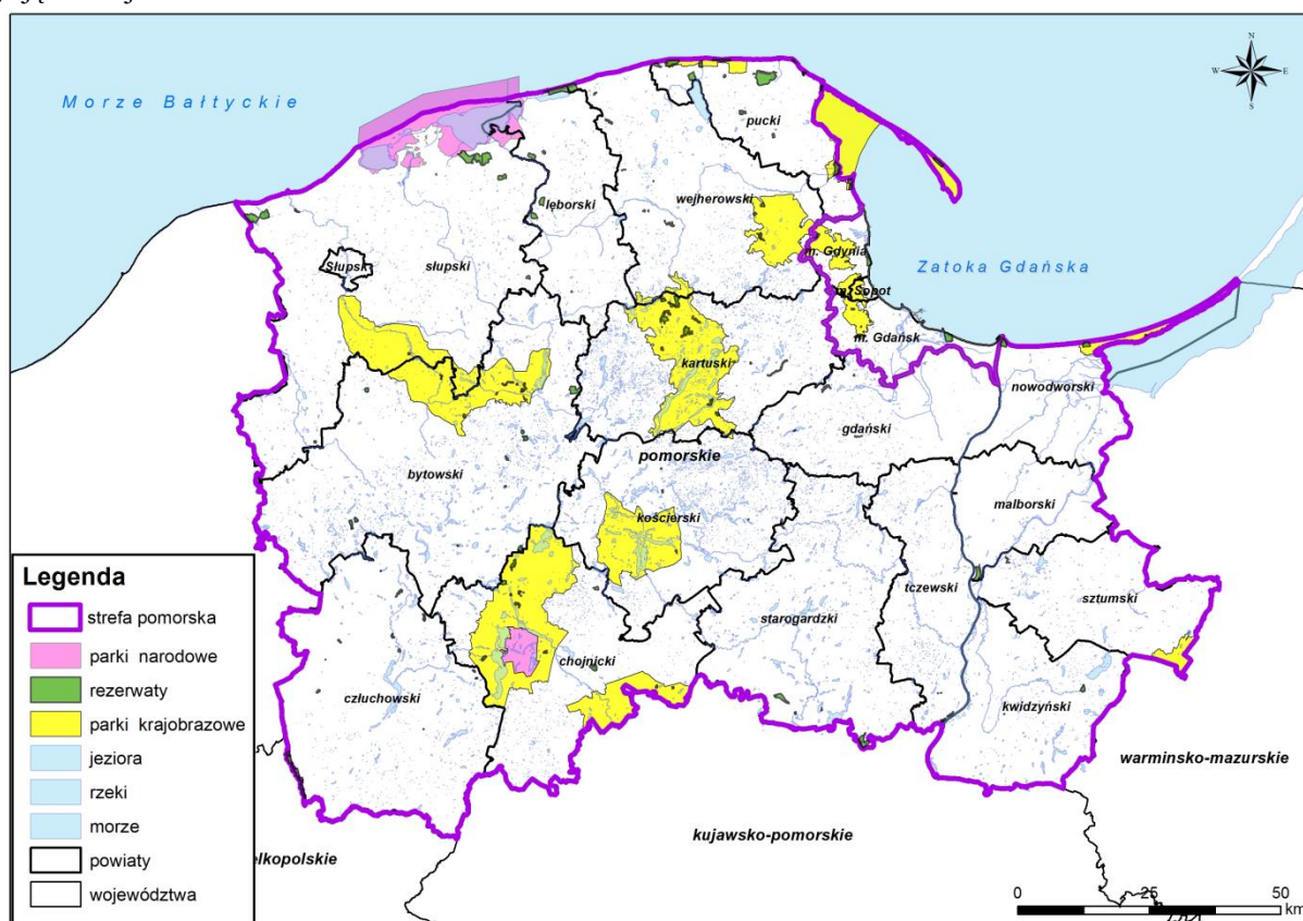
Rysunek 5. Formy ochrony przyrody w województwie pomorskim 4
