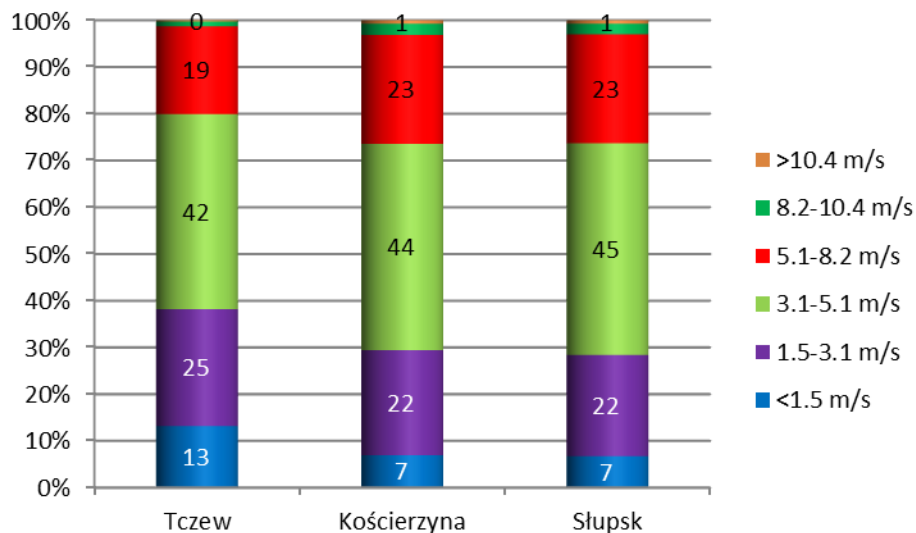
Rysunek 49. Procentowy rozkład prawdopodobieństwa występowania prędkości wiatru w określonych przedziałach na wybranych stanowiskach w województwie pomorskim w 2013 r.
