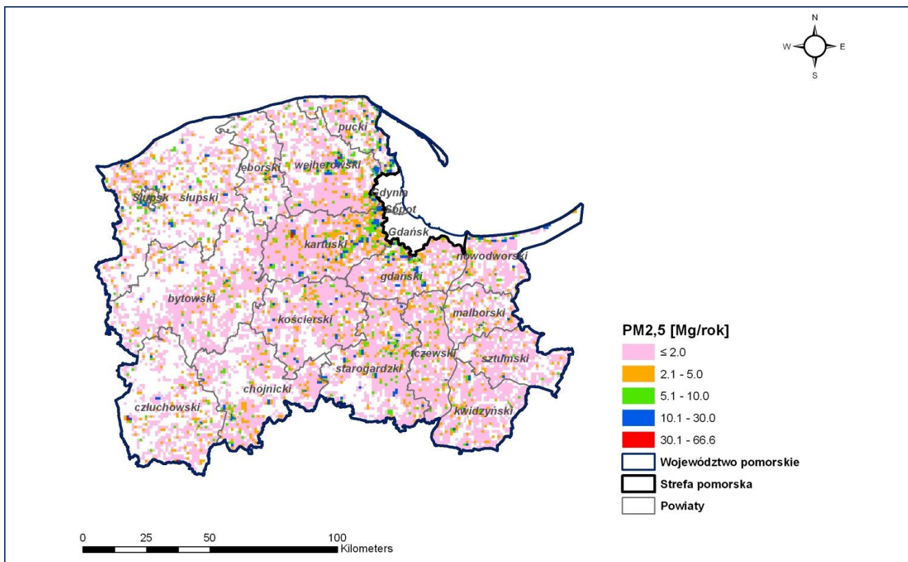
Rysunek 16. Emisja powierzchniowa pyłu zawieszonego PM_{2,5} z terenu strefy pomorskiej w 2013 r.
