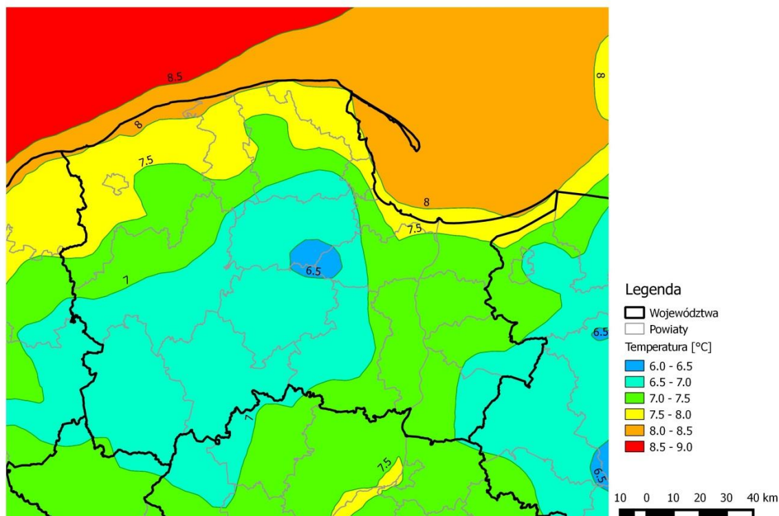
Rysunek 44. Rozkład średniej rocznej wartości temperatury powietrza [°C]
