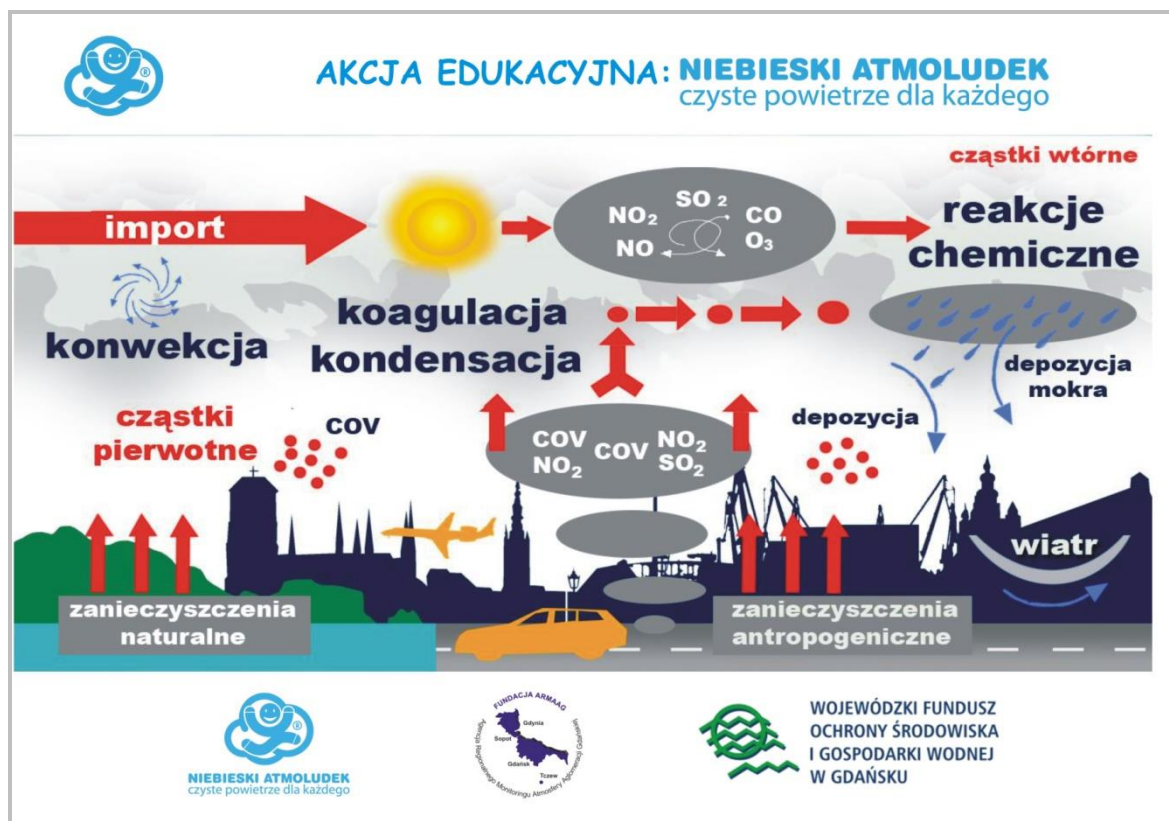
Rysunek 6. Powstawanie pyłu zawieszonego
