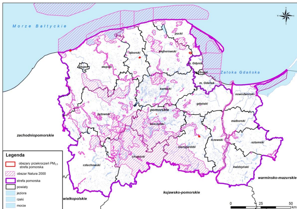
Rysunek 42. Mapa obszarów zagrożeń na tle obszarów NATURA 2000
