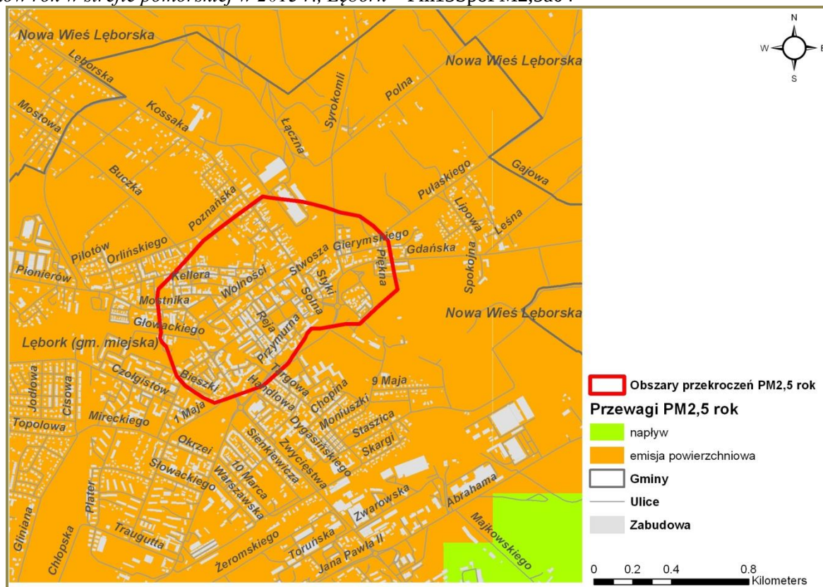
Rysunek 34. Przeważający typ emisji w stężeniach pyłu zawieszonego PM_{2,5} o okresie uśredniania wyników rok w strefie pomorskiej w 2013 r., Lębork – Pm13SpoPM2,5a04
