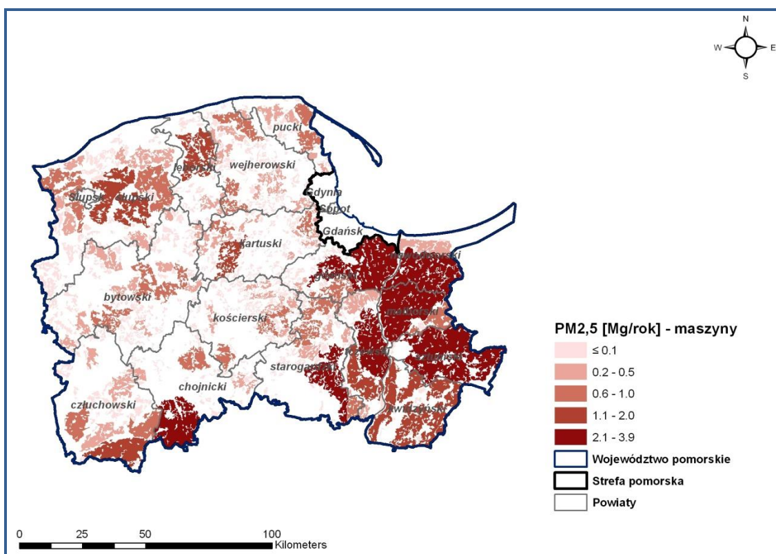
Rysunek 22. Emisja pyłu zawieszonego PM_{2,5} z rolnictwa (maszyny rolnicze) z terenu strefy pomorskiej w 2013r.
