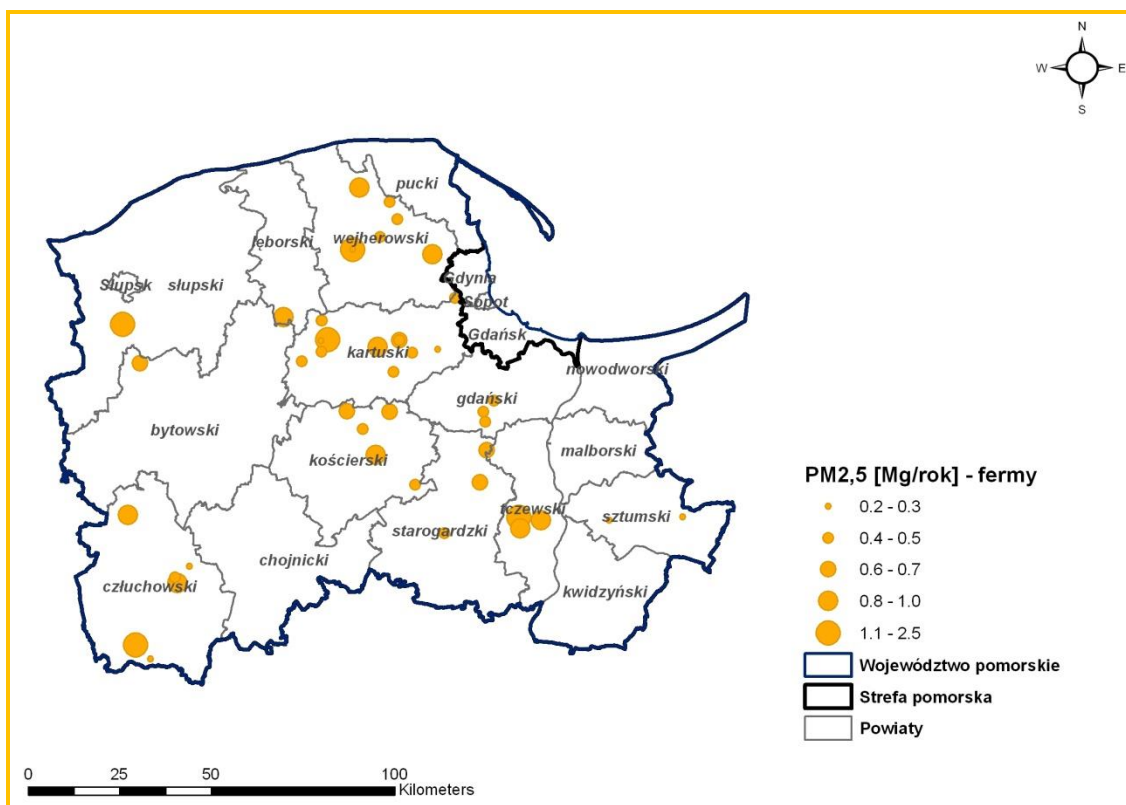
Rysunek 19. Emisja pyłu zawieszonego PM_{2,5} z rolnictwa (fermy) z terenu strefy pomorskiej w 2013 r.
