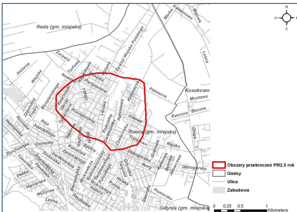
Rysunek 29. Obszar przekroczeń poziomu dopuszczalnego pyłu zawieszonego PM_{2,5} o okresie uśredniania wyników rok w strefie pomorskiej w 2013 r., Rumia – PM13SpoPM2,5a02
