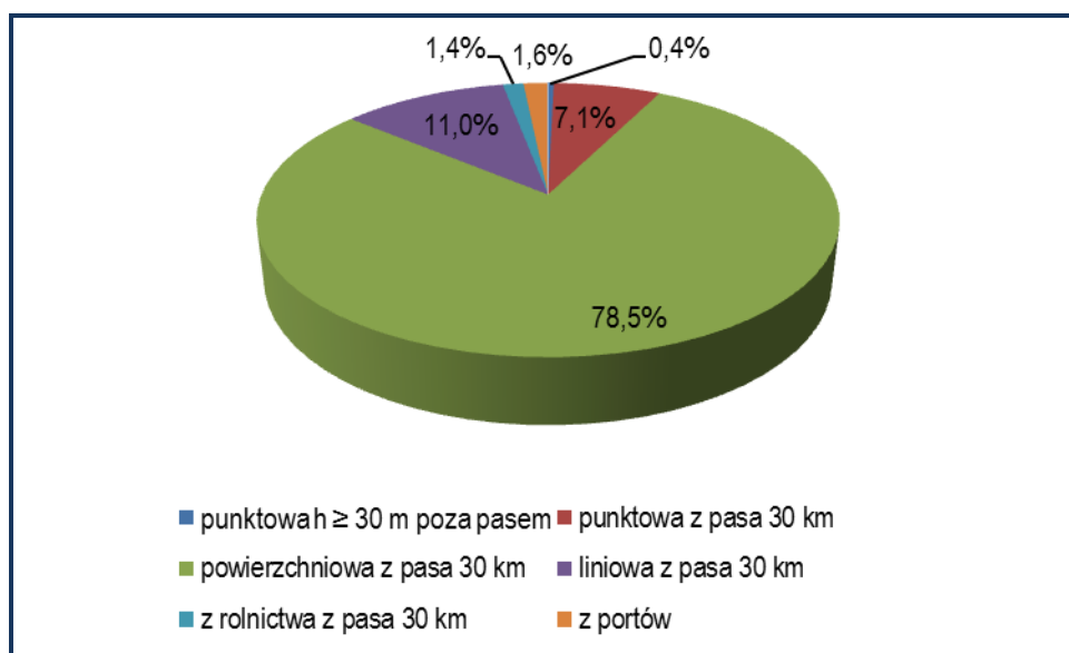
Rysunek 12. Udział procentowy emisji napływowej pyłu zawieszonego PM_{2,5} dla strefy pomorskiej w 2013r.
