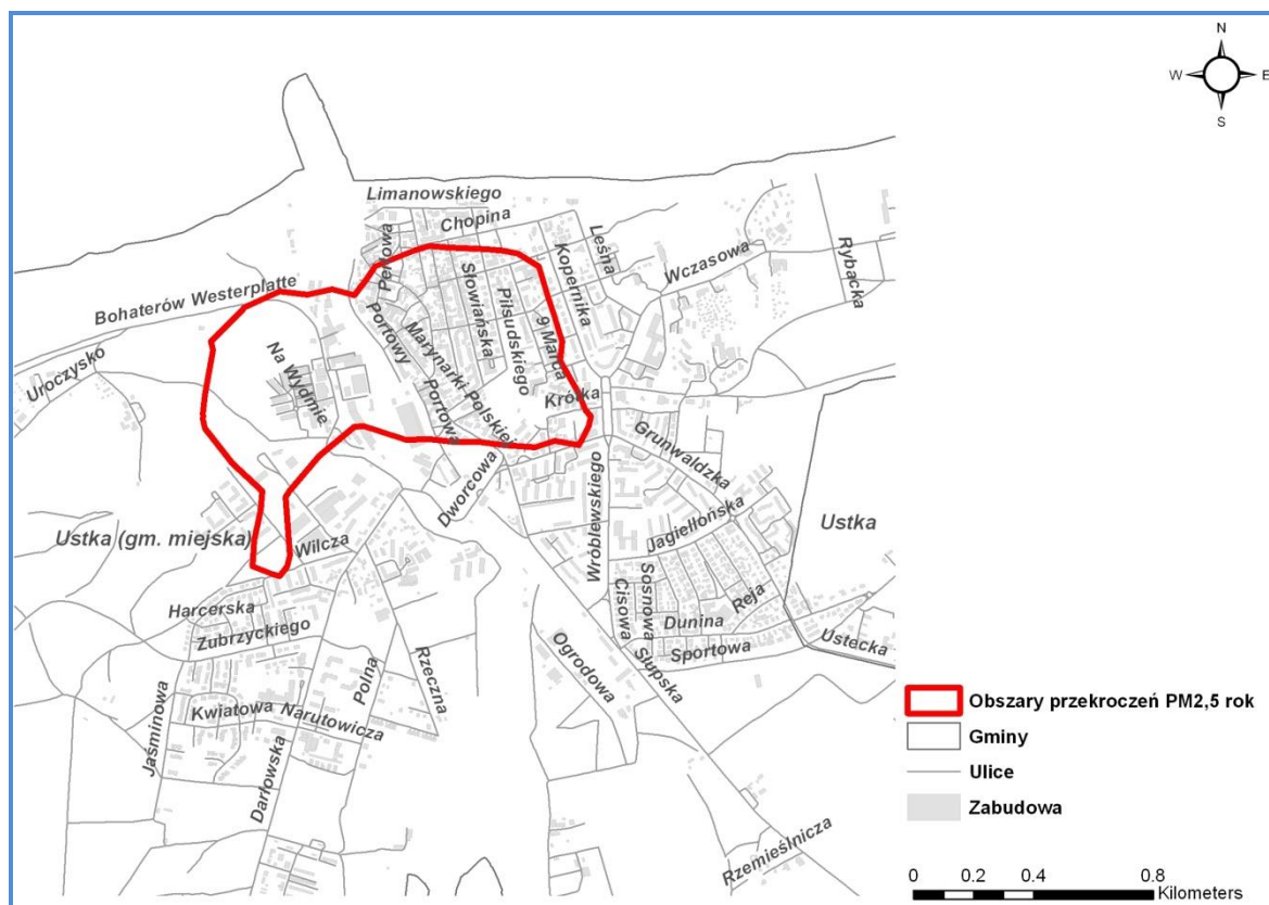
Rysunek 35. Obszar przekroczeń poziomu dopuszczalnego pyłu zawieszonego PM_{2,5} o okresie uśredniania wyników rok w strefie pomorskiej w 2013 r., Ustka – Pm13SpoPM2,5a04
