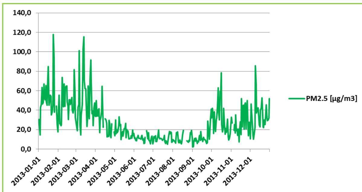
Rysunek 38. Roczny przebieg średnich dobowych wartości pyłu zawieszonego PM_{2,5} na stanowisku pomiarowym w Kościerzynie, w strefie pomorskiej w 2013 r.
