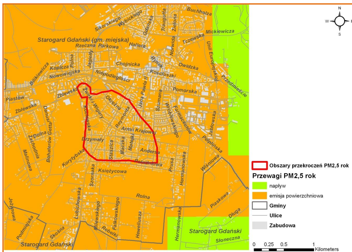
Rysunek 32. Przeważający typ emisji w stężeniach pyłu zawieszonego PM_{2.5} o okresie uśredniania wyników rok w strefie pomorskiej w 2013 r., Starogard Gdański – Pm13Spo PM_{2.5} a03
