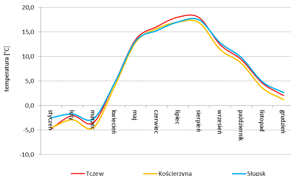
Rysunek 45. Przebieg średnich miesięcznych wartości temperatury powietrza na wybranych stanowiskach w województwie pomorskim w 2013 r.
