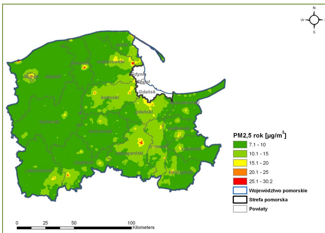
Rysunek 25. Stężenia pyłu zawieszonego PM_{2,5} o okresie uśredniania wyników rok w strefie pomorskiej pochodzące z łącznej emisji wszystkich typów w 2013 r.
