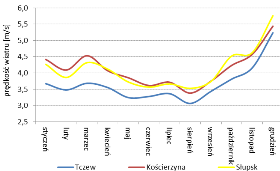
Rysunek 47. Średnia miesięczna wartość prędkości wiatru [m/s] na wybranych stanowiskach w województwie pomorskim w 2013 r.
