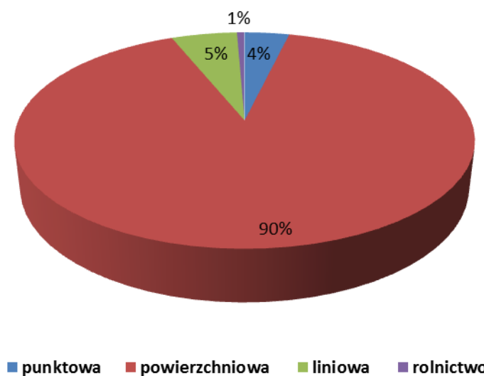
Rysunek 13. Udział procentowy emisji pyłu zawieszonego PM_{2,5} dla strefy pomorskiej w 2013 r.
