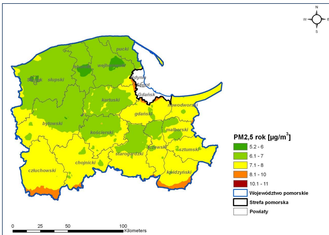
Rysunek 24. Stężenia pyłu zawieszonego PM_{2,5} o okresie uśredniania wyników rok w strefie pomorskiej pochodzące z tła całkowitego w 2013 r.
