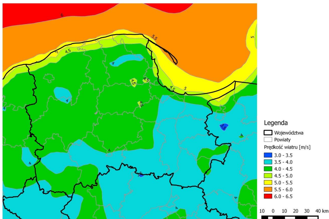
Rysunek 46. Rozkład średniej rocznej wartości prędkości wiatru [m/s] w województwie pomorskim w 2013 r.
