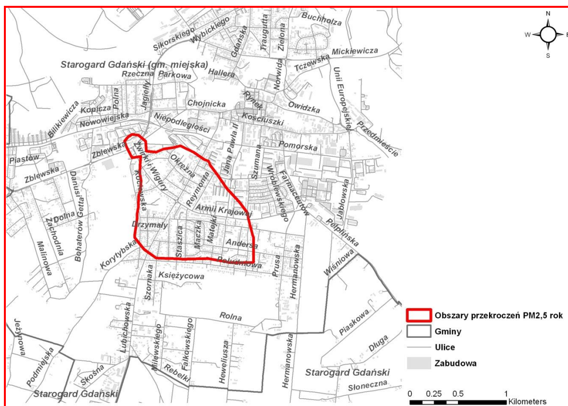
Rysunek 31. Obszar przekroczeń poziomu dopuszczalnego pyłu zawieszonego PM_{2.5} o okresie uśredniania wyników rok w strefie pomorskiej w 2013 r., Starogard Gdański – Pm13Spo PM_{2.5} a03
