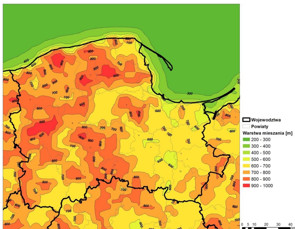
Rysunek 56. Rozkład średniej rocznej wartości wysokości warstwy mieszaniny [m] w województwie pomorskim w 2013 r.
