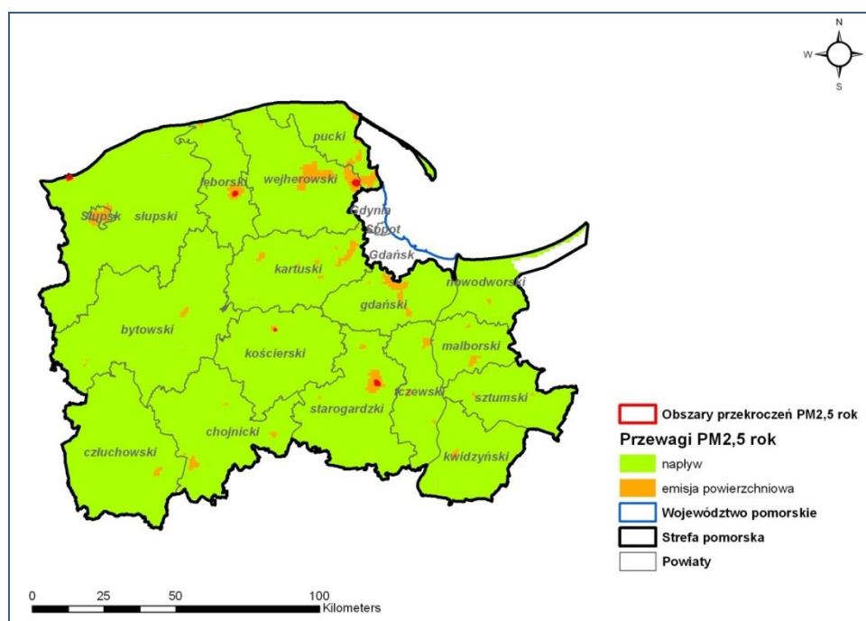
Rysunek 26. Przewagi poszczególnych typów emisji w stężeniach całkowitych pyłu zawieszonego PM_{2,5} o okresie uśredniania wyników rok w strefie pomorskiej w 2013 r.
