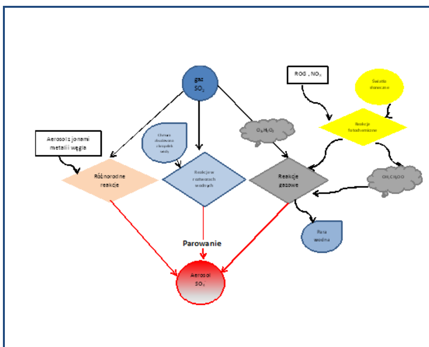
Rysunek 9. Procesy utleniania dwutlenku siarki w atmosferze wykorzystane w mechanizmie MESOPUFF II w modelu CALPUFF (źródło: A User's Guide for the CALPUFF Dispersion Model)
