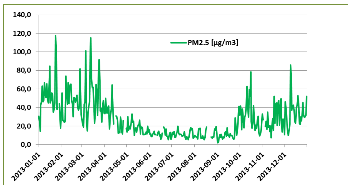
Rysunek 7. Przebieg zmian stężenia pyłu PM_{2,5} w roku 2013 na podstawie danych stacji w Kościerzynie
