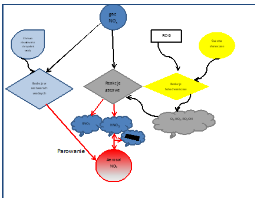
Rysunek 10. Procesy utleniania tlenków azotu w atmosferze wykorzystane w mechanizmie MESOPUFF II w modelu CALPUFF (źródło: A User's Guide for the CALPUFF Dispersion Model)
