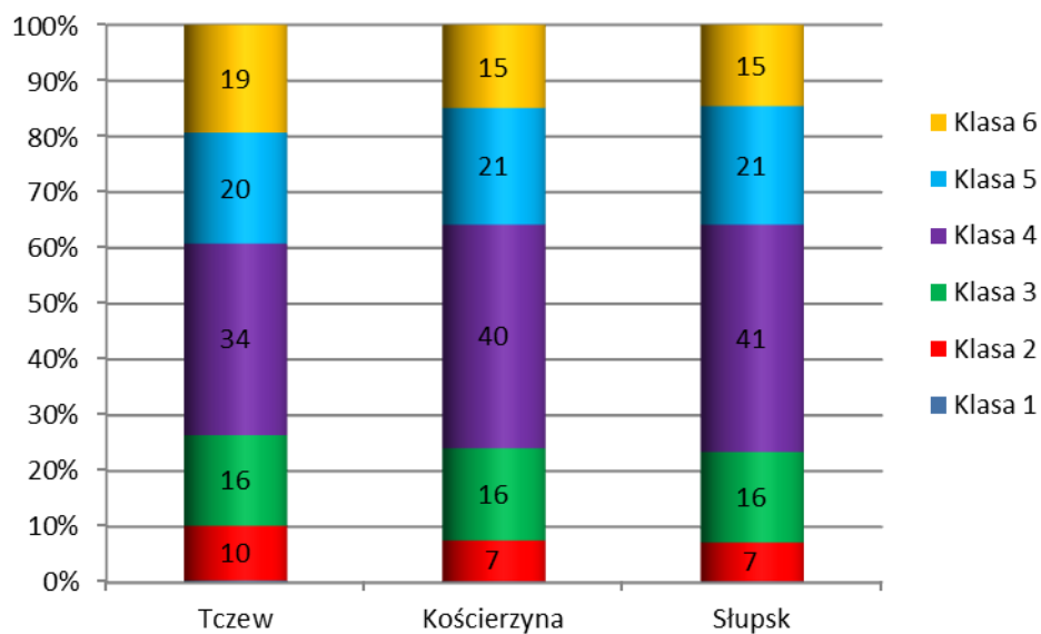
Rysunek 57. Rozkład prawdopodobieństwa występowania klas równowagi atmosfery na wybranych stanowiskach w województwie pomorskim w 2013 r.
