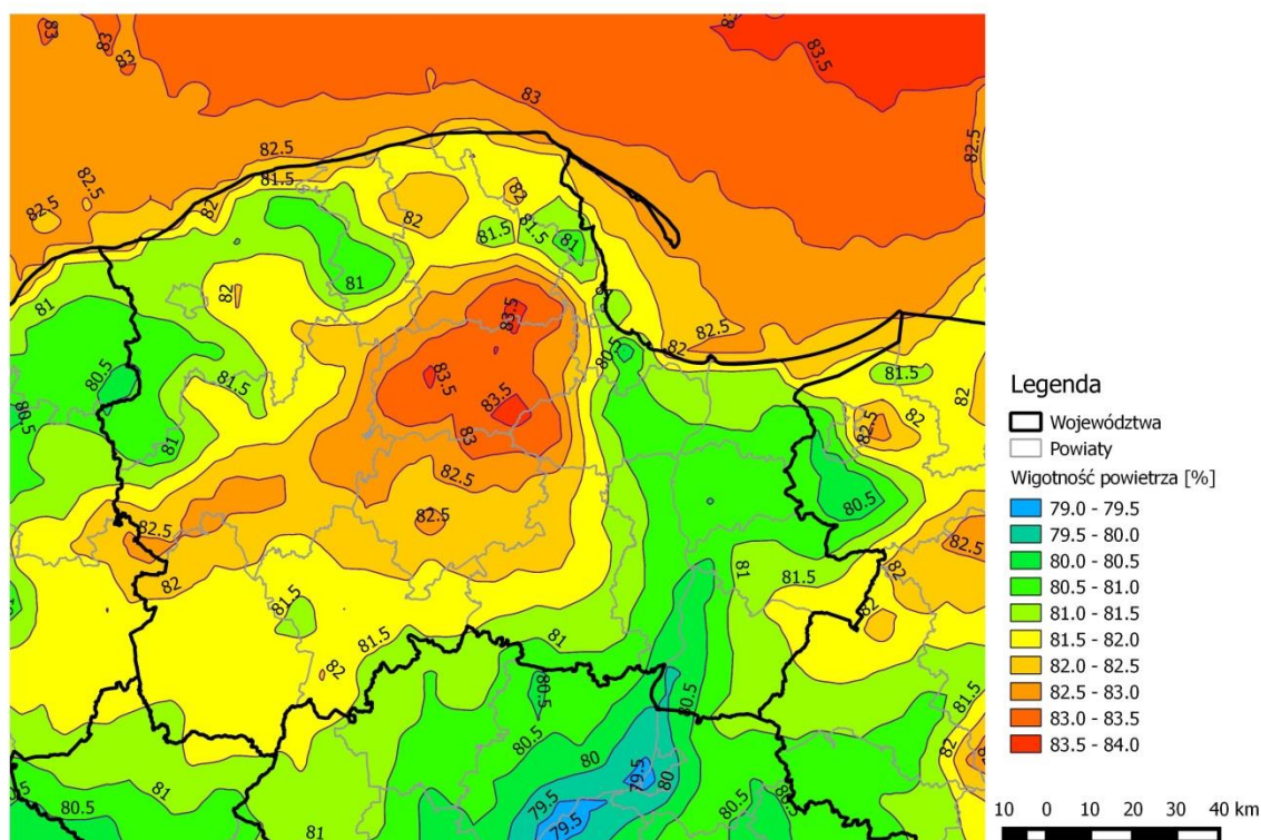
Rysunek 54. Rozkład średniej rocznej wartości wilgotności względnej powietrza [%] w województwie pomorskim w 2013r.
