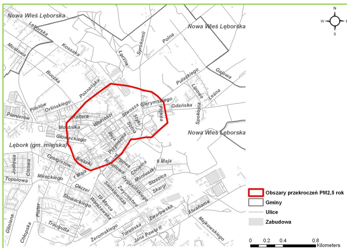
Rysunek 33. Obszar przekroczeń poziomu dopuszczalnego pyłu zawieszonego PM_{2,5} o okresie uśredniania wyników rok w strefie pomorskiej w 2013 r., Lębork – Pm13SpoPM2,5a04
