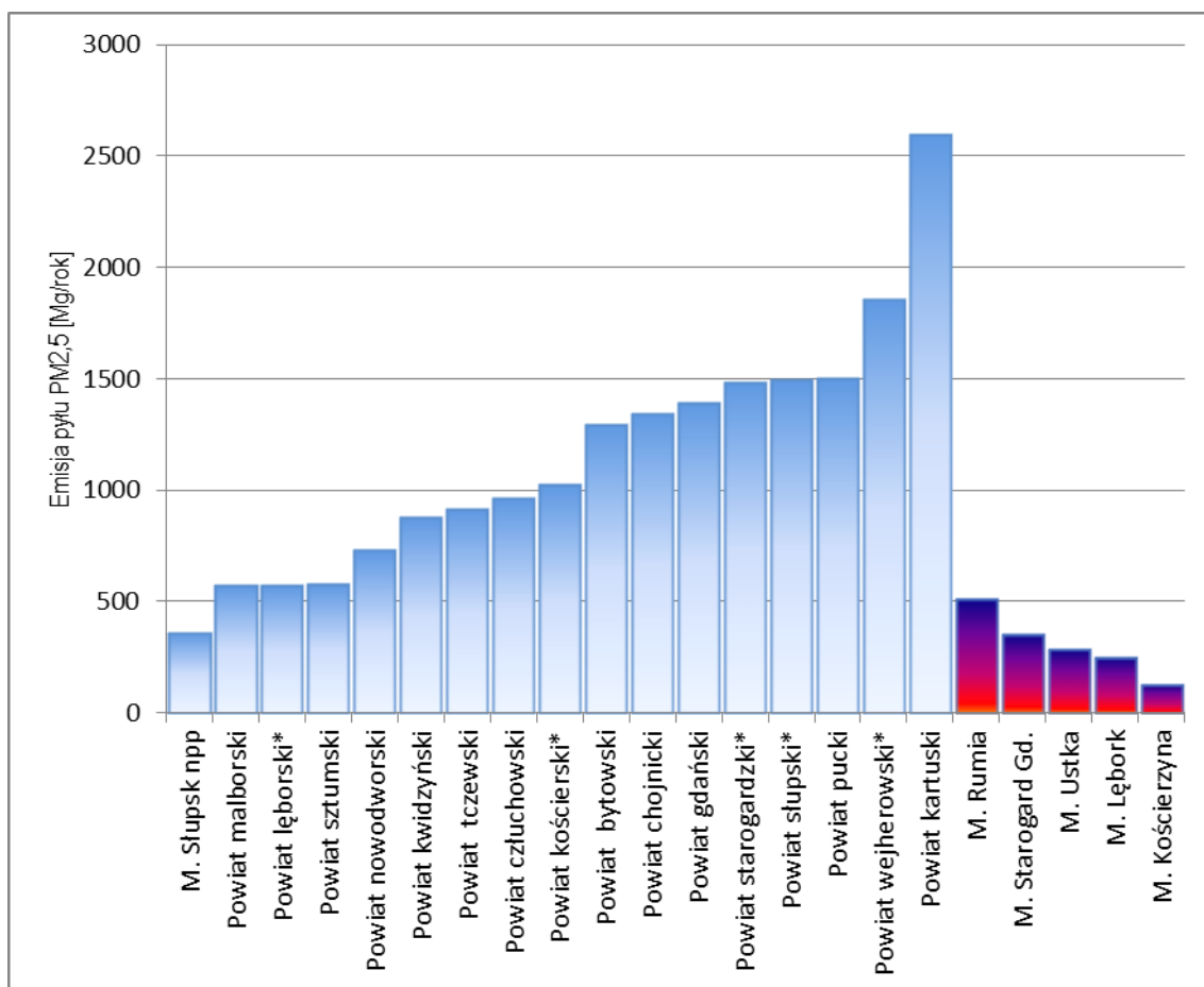
Rysunek 14. Emisja powierzchniowa pyłu PM_{2,5} [Mg] w strefie pomorskiej w roku 2013
