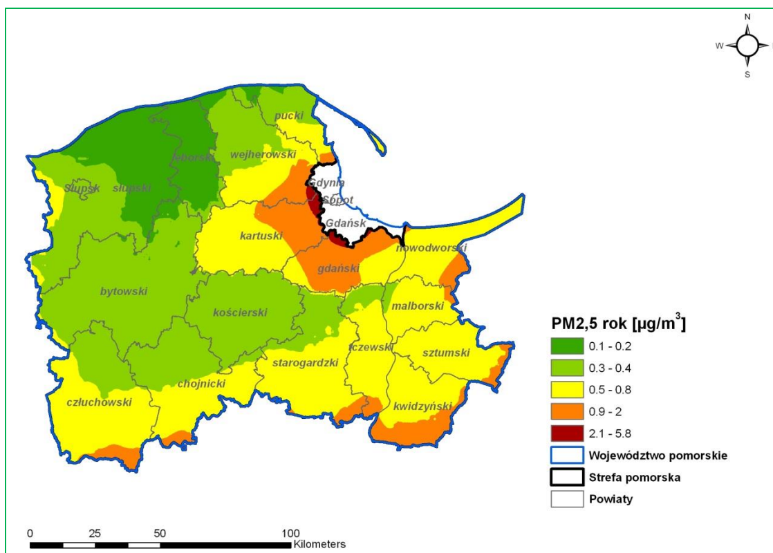
Rysunek 23. Stężenia pyłu zawieszonego PM_{2,5} o okresie uśredniania wyników rok w strefie pomorskiej pochodzące z tła regionalnego w 2013 r.
