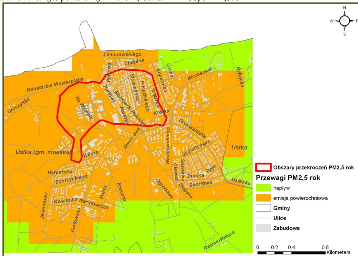
Rysunek 36. Przeważający typ emisji w stężeniach pyłu zawieszonego PM_{2,5} o okresie uśredniania wyników rok w strefie pomorskiej w 2013 r., Ustka – Pm13SpoPM2,5a04
