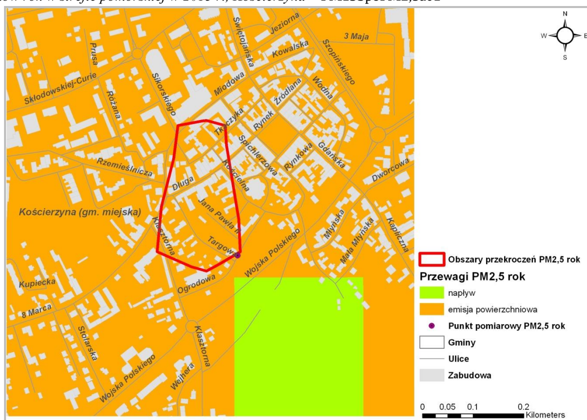
Rysunek 28. Przeważający typ emisji w stężeniach pyłu zawieszonego PM_{2.5} o okresie uśredniania wyników rok w strefie pomorskiej w 2013 r., Kościerzyna – PM13SpoPM2,5a01
