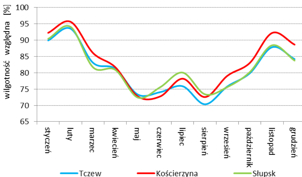
Rysunek 55. Przebieg średnich miesięcznych wartości wilgotności względnej powietrza [%] na wybranych stanowiskach w województwie pomorskim w 2013 r.
