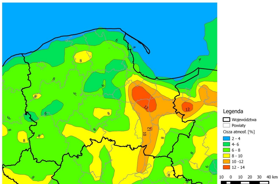
Rysunek 48. Rozkład częstości występowania cisz atmosferycznych w województwie pomorskim w 2013r.
