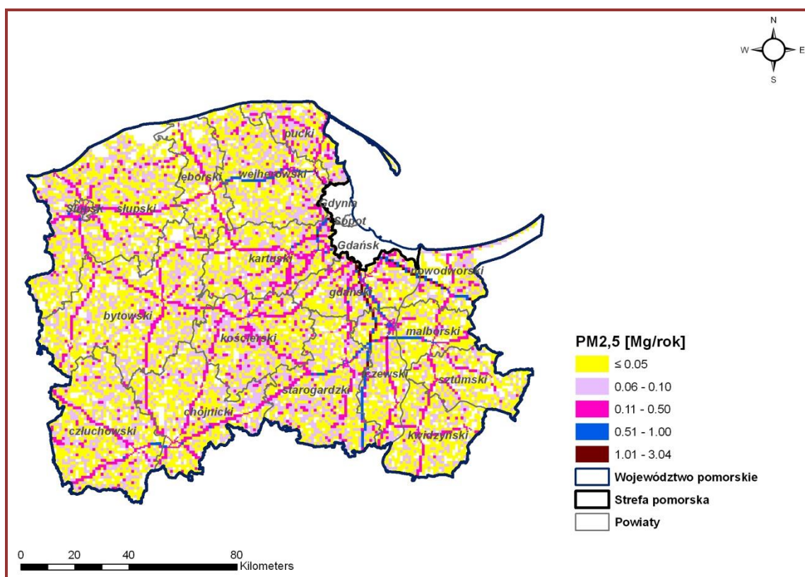
Rysunek 17. Emisja liniowa pyłu zawieszonego PM 2,5 z terenu strefy pomorskiej w 2013 r.
