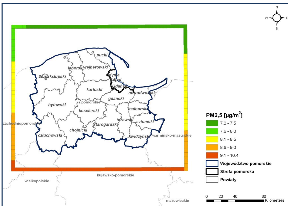
Rysunek 11. Warunki brzegowe pyłu zawieszonego PM_{2,5} dla strefy pomorskiej w 2013 r.
