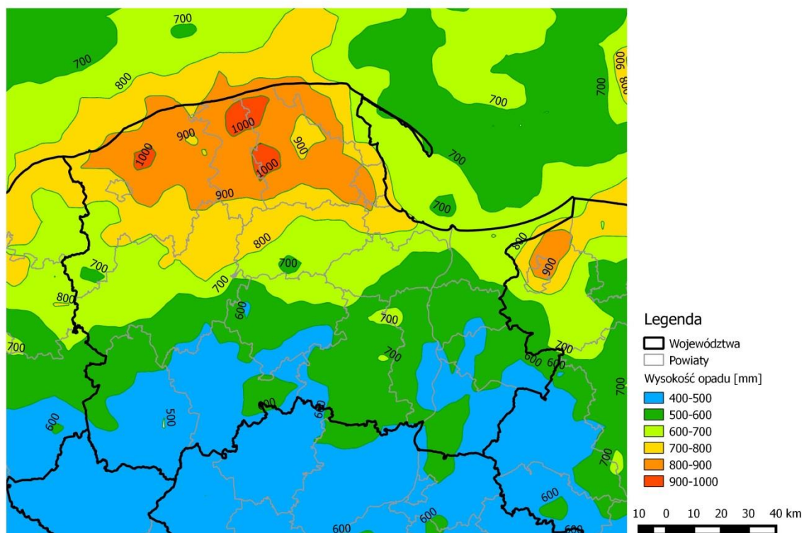
Rysunek 52. Rozkład rocznej sumy opadów atmosferycznych [mm] w województwie pomorskim w 2013r.
